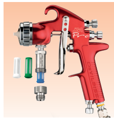
Accessoire en option, kit filtre inox VSA-512 (avec 3 éléments)
