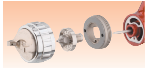
Taille (mm) des buses et aiguilles du pistolet JGA Pro pression : 0.85, 1.0, 1.2, 1.4, 1.6, 1.8 Taille (mm) des buses et aiguilles du pistolet JGA Pro suction : 1.4, 1.6, 1.8 Taille (mm) des buses et aiguilles du pistolet GFG Pro gravité : 1.4, 1.6, 1.8
